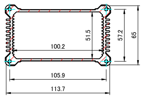
A-A ( 1 : 2.5 )
