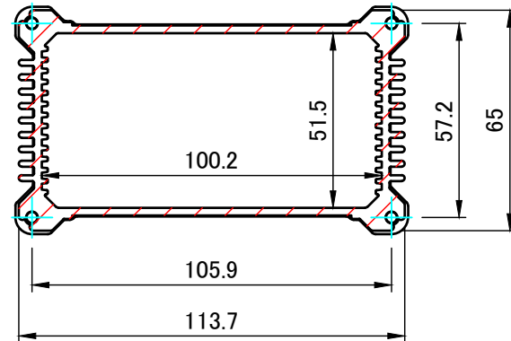
A-A (1:2)
