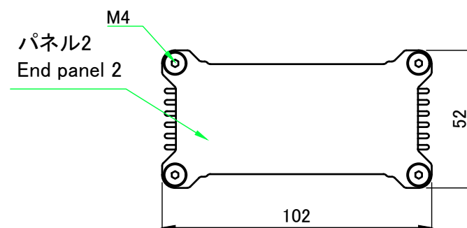
A-A ( 1 : 2 )
