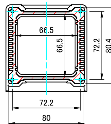
A-A (1:2.5)
