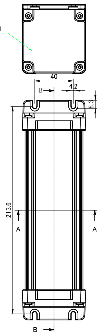
フランジ付側板1 Flanged end panel 1
