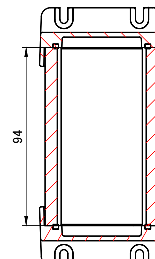
C-C (1:2)
