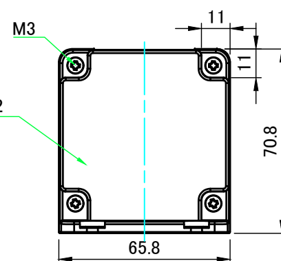
A-A (1:2)
