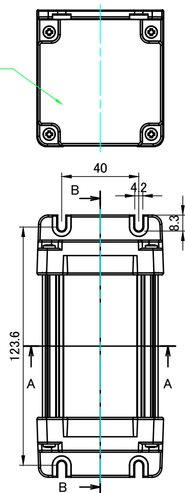
フランジ付側板1 Flanged end panel 1
