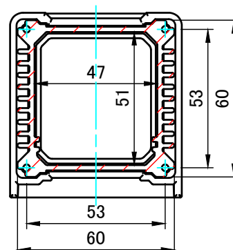
A-A (1:2)
