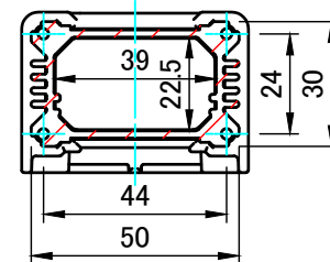
A-A (1:2)
