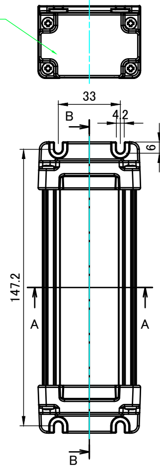
フランジ付側板1 Flanged end panel 1
