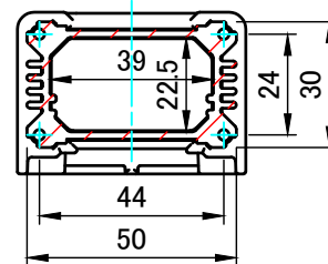
A-A (1:2)
