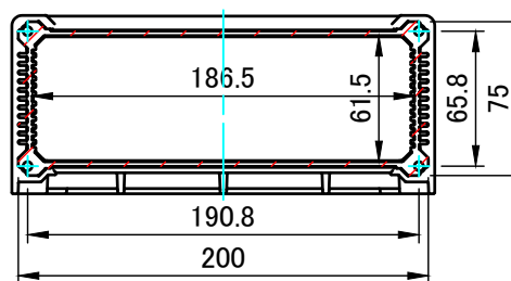
A-A (1:4)
