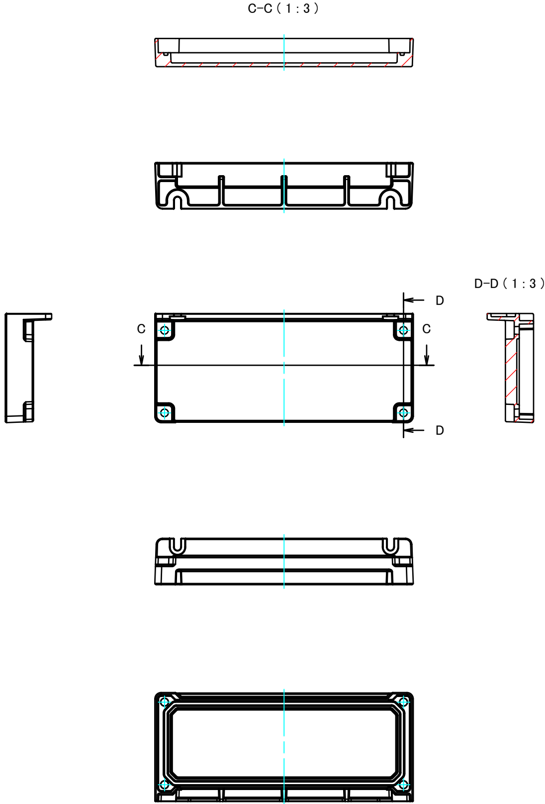
フランジ付側板2 Flanged end panel 2
