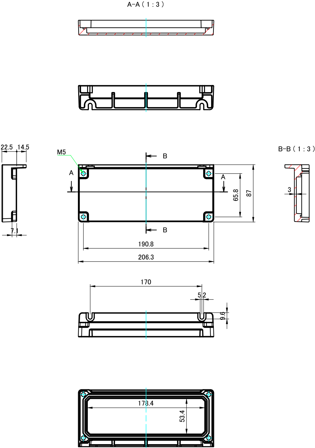
フランジ付側板1 Flanged end panel 1
