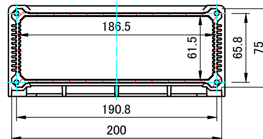
A-A ( 1 : 3.5 )
