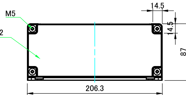
A-A ( 1 : 3.5 )
