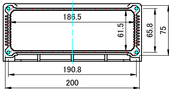
A-A ( 1 : 3.5 )
