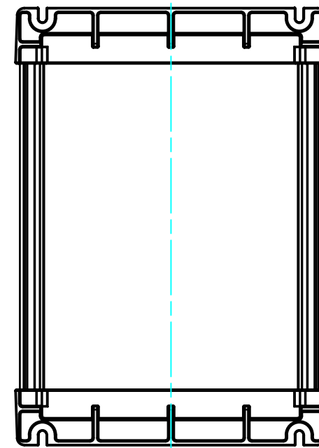
C-C ( 1 : 3.5 )
