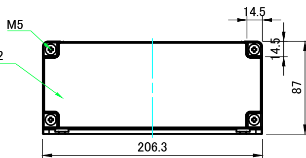
A-A ( 1 : 3.5 )
