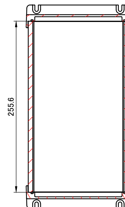
C-C ( 1 : 3.5 )
