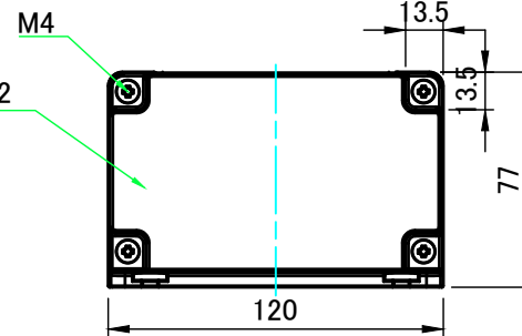
A-A (1:3)
