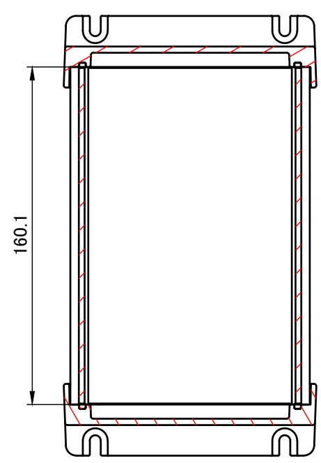
C-C ( 1 : 2.5 )
