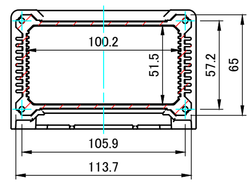
A-A ( 1 : 2.5 )
