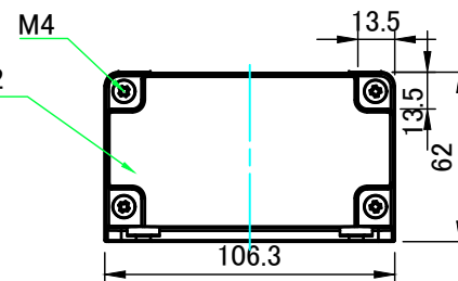
フランジ付側板2 Flanged end panel 2
