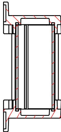
B-B (1:2.5)
