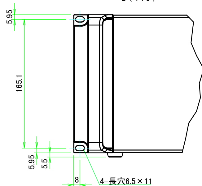
D ( 1 : 3 )
