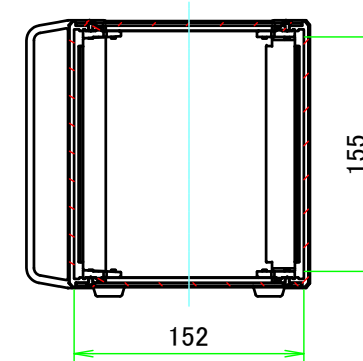
A-A ( 1 : 5 )
