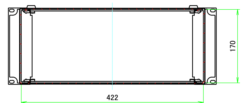
C-C ( 1 : 5 )
