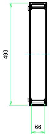
A-A (1:8)
