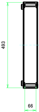
A-A (1:8)
