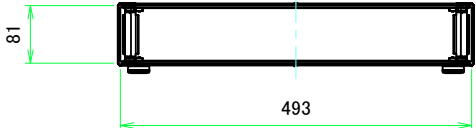
B-B ( 1 : 7.5 )
