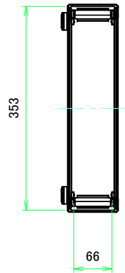
A-A (1 : 6.5)
