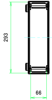
A-A (1 : 6.5)
