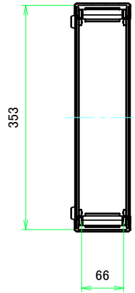
A-A (1:6)
