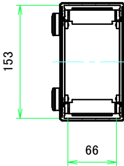
A-A (1:5)
