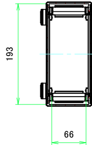
A-A (1:5)
