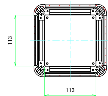
C-C (1:3.5)
