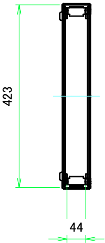
A-A ( 1:8.5 )
