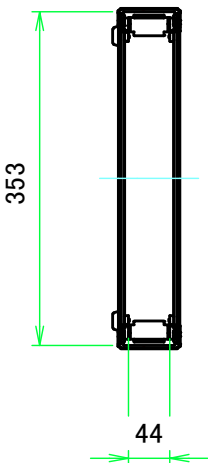
A-A ( 1:8 )
