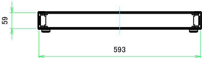
B-B ( 1:8 )
