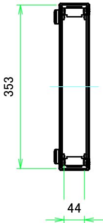
A-A ( 1:8 )
