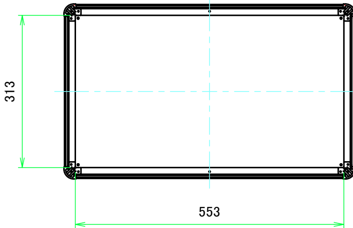
C-C ( 1:8 )
