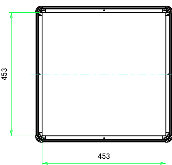
C-C ( 1:8 )
