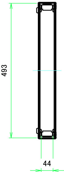
A-A ( 1:8 )
