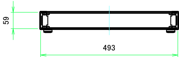
B-B ( 1:8 )
