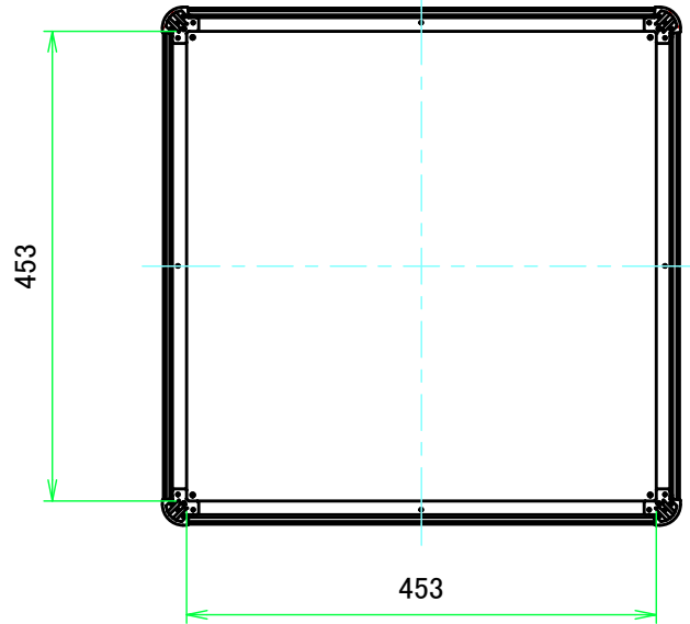
C-C ( 1:8 )
