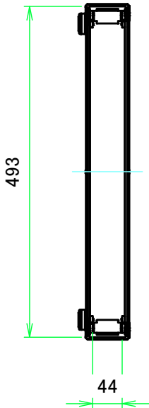
A-A ( 1:8 )
