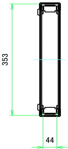
A-A ( 1:7 )
