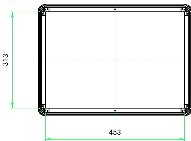
C-C ( 1:7 )
