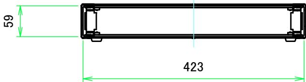
B-B ( 1:7 )
