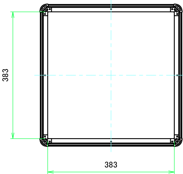
C-C ( 1:7 )
