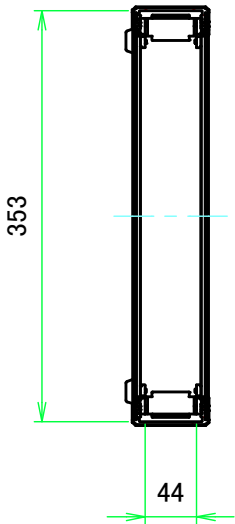
A-A ( 1:6.5 )
