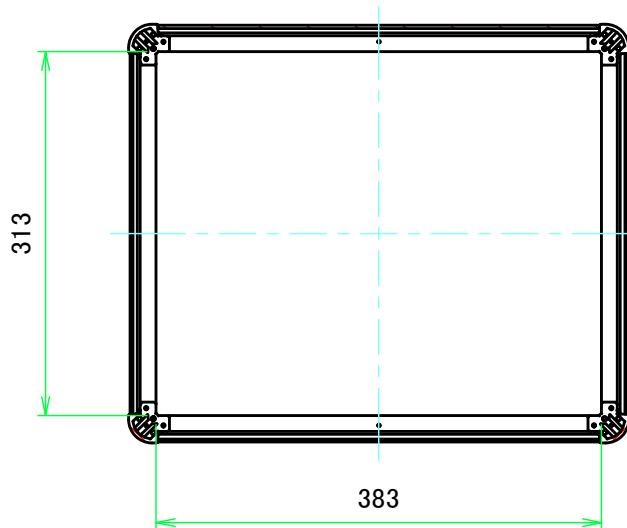
C-C ( 1:6.5 )
