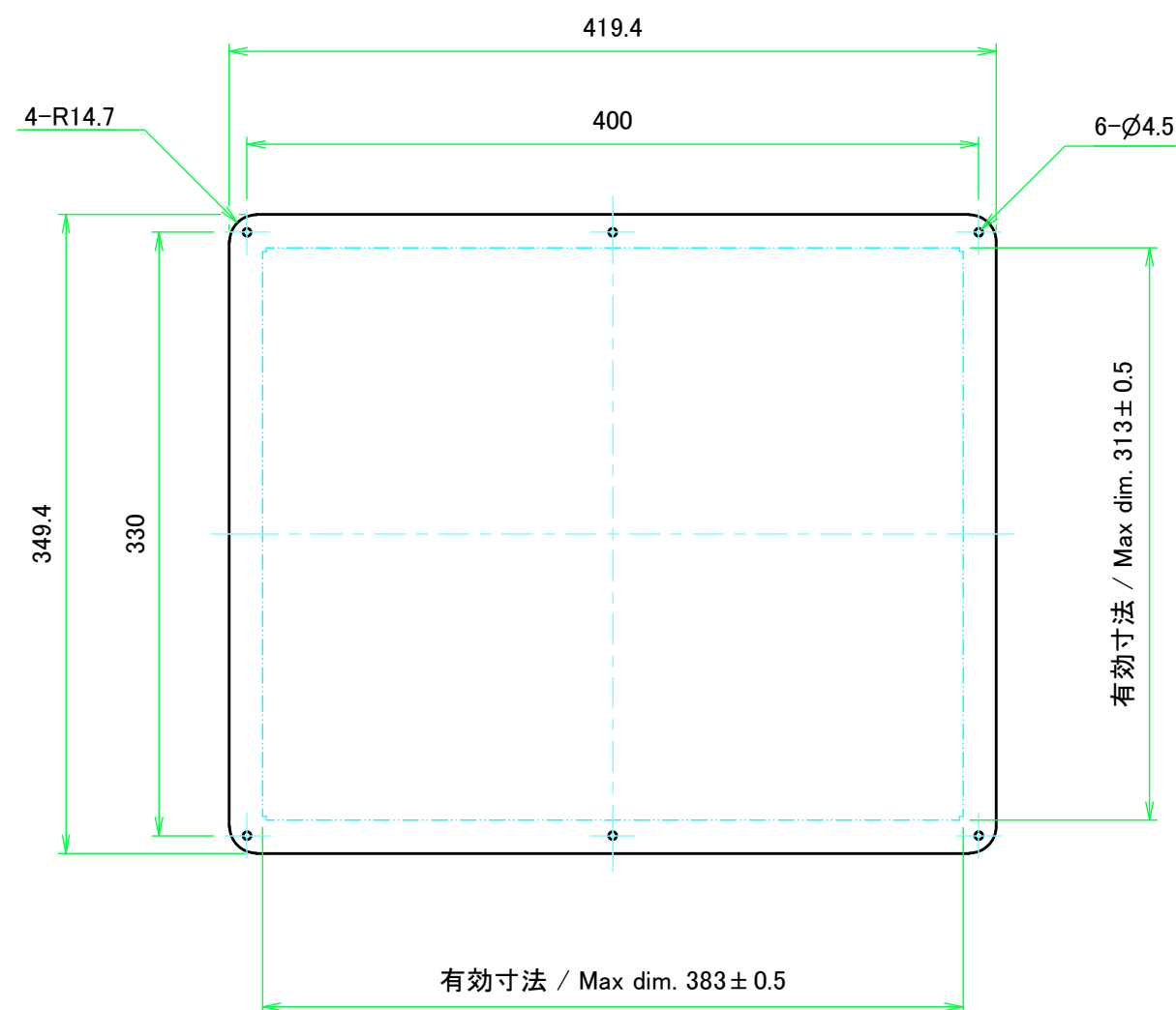
保護シート側 Surface protective film side
