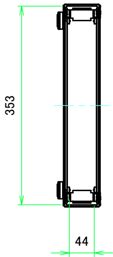
A-A ( 1:6.5 )
