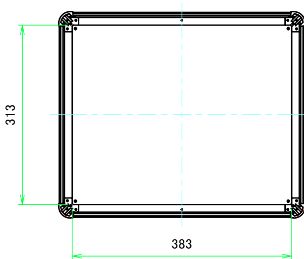
C-C ( 1:6.5 )
