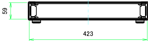
B-B ( 1:6.5 )
