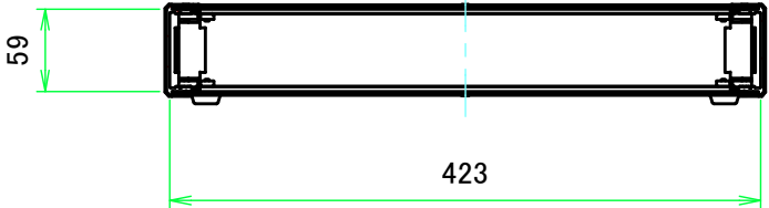
B-B ( 1:6 )
