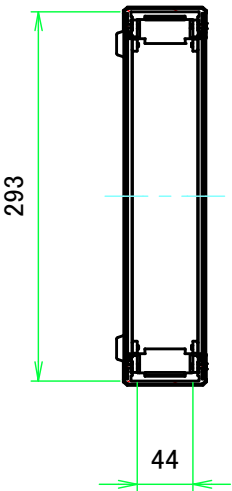
A-A ( 1:6 )
