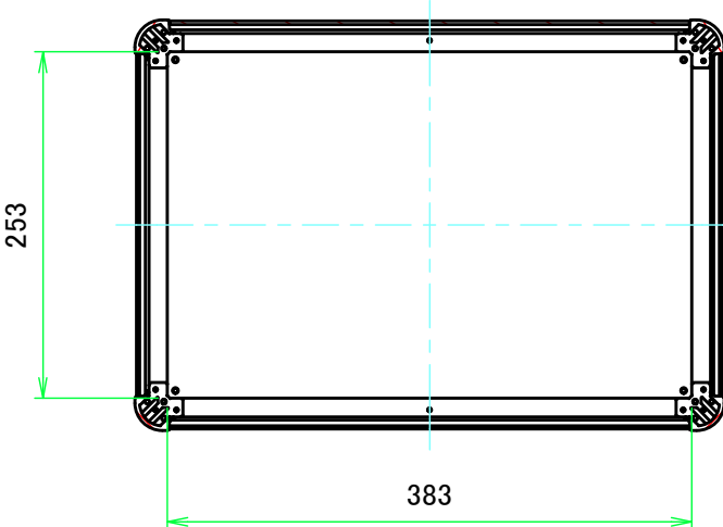
C-C ( 1:6 )
