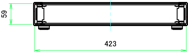
B-B ( 1:6 )
