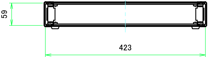
B-B ( 1:6 )
