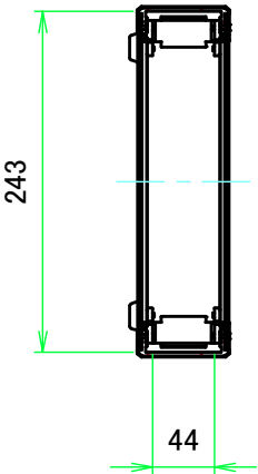
A-A ( 1:6 )
