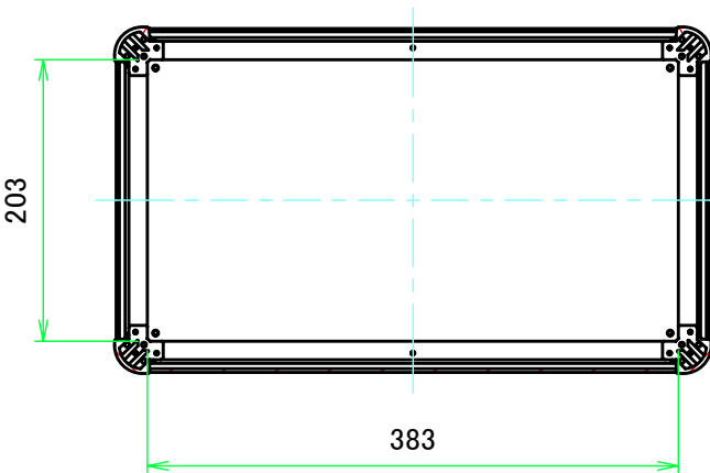
C-C ( 1:6 )
