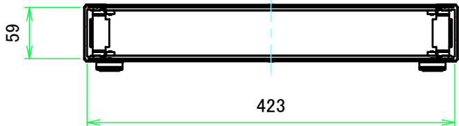
B-B ( 1:6 )
