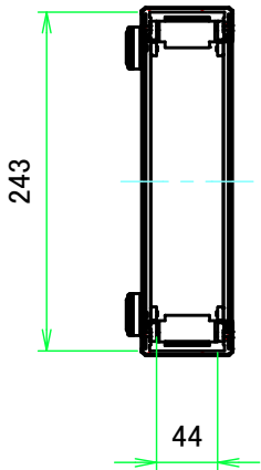
A-A ( 1:6 )
