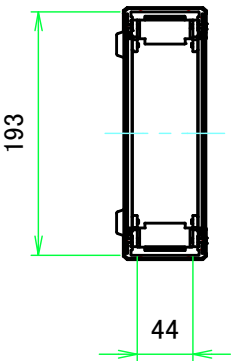
A-A ( 1:6 )
