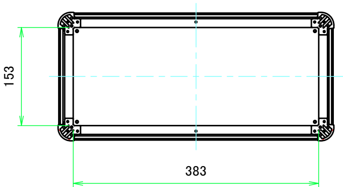
C-C ( 1:6 )
