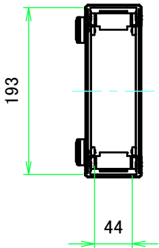
A-A ( 1:6 )
