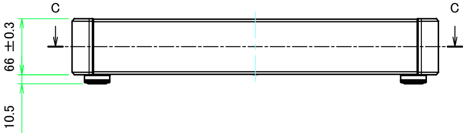
B-B ( 1 : 4.5 )
