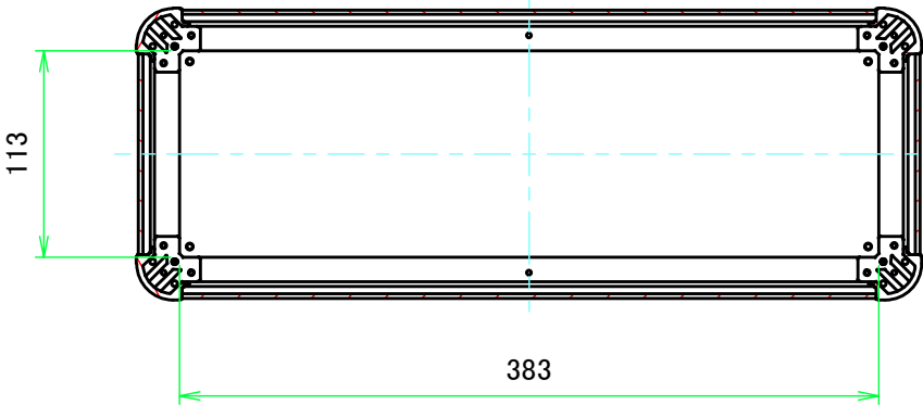
C-C ( 1 : 4.5 )
