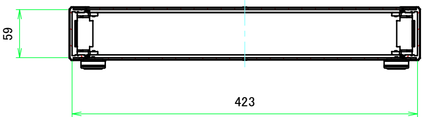
B-B ( 1 : 4.5 )
