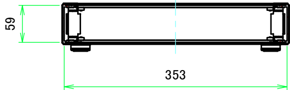
B-B ( 1:6 )
