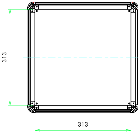
C-C ( 1:6 )
