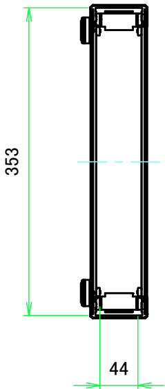
A-A ( 1:6 )
