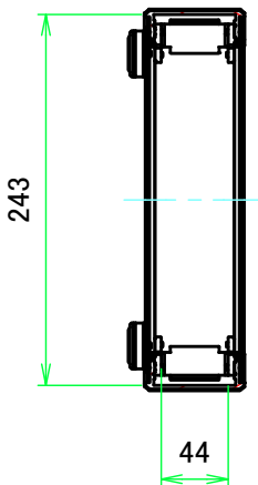
A-A ( 1:5.5 )
