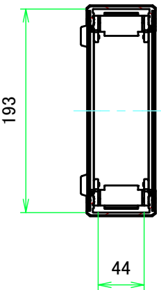
A-A ( 1:5 )
