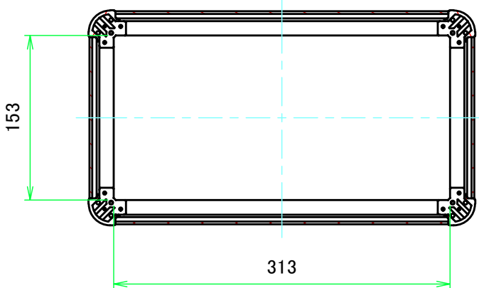
C-C ( 1:5 )
