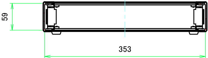
B-B ( 1:5 )
