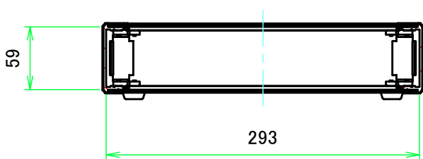
B-B ( 1:5 )
