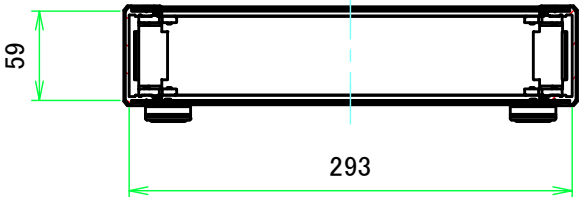
B-B ( 1:5 )
