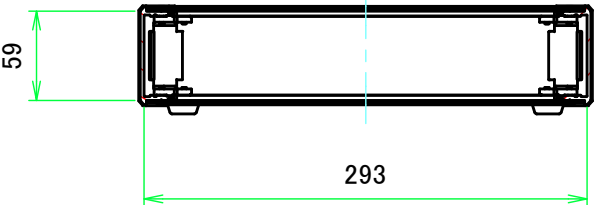
B-B ( 1:5 )
