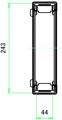
A-A ( 1:5 )
