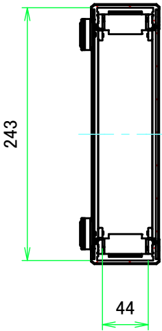
A-A ( 1:5 )
