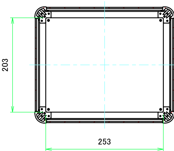
C-C ( 1:5 )
